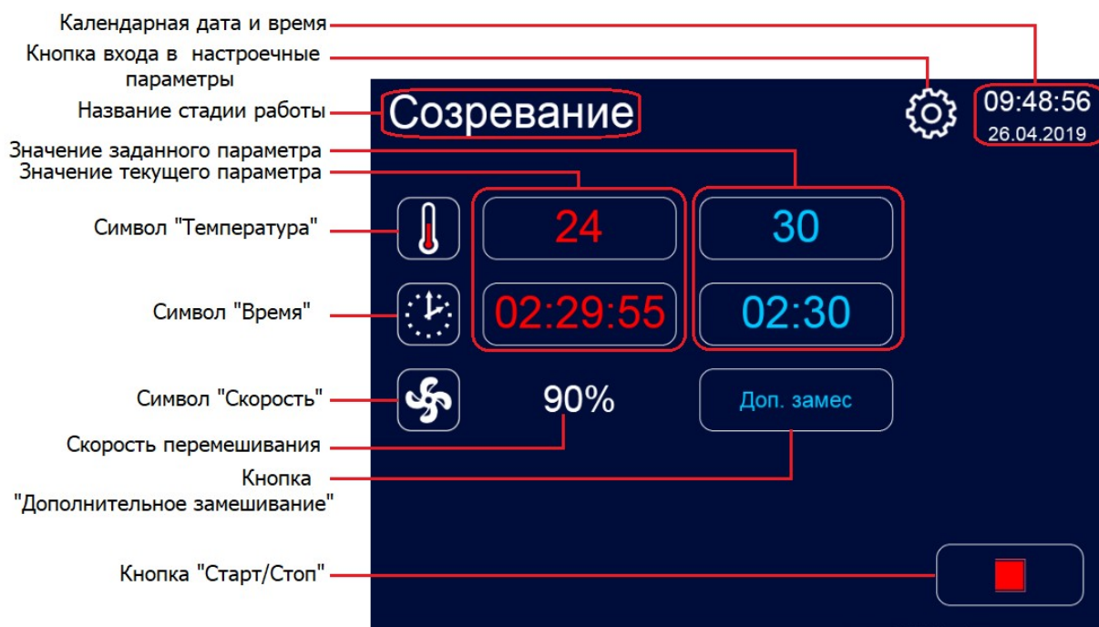
Рисунок 6 Описание экрана
